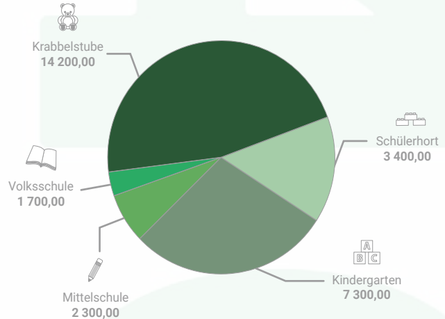
Kosten pro Kind und Jahr laut vorläufigem Budget 2025
